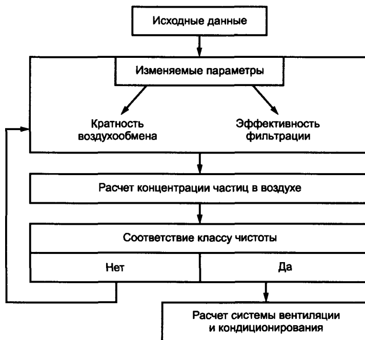
Рисунок С.2 - Подбор кратности воздухообмена в зависимости от класса чистоты и эффективности фильтрации воздуха
