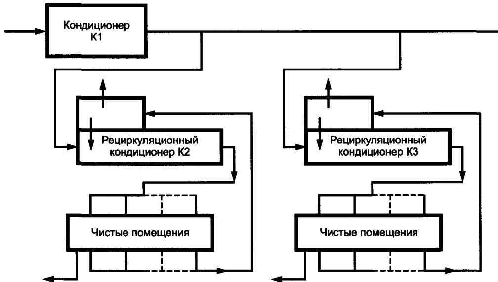
Рисунок А.4 - Двухуровневая система вентиляции и кондиционирования
