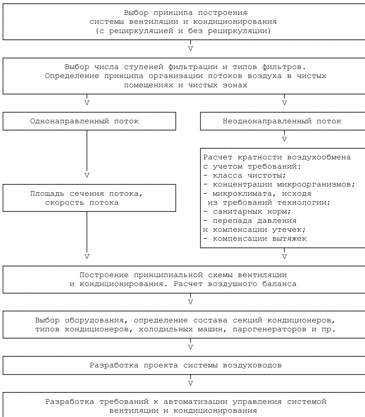
Рисунок В.2 - Последовательность разработки проектных решений по вентиляции и кондиционированию
