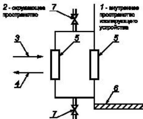
Рисунок D.4 — Передаточное устройство типа В2
