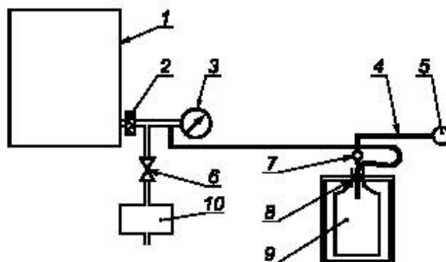
1 — изолирующее устройство; 2 — НЕРА фильтр (опция); 3 — манометр; 4 — резиновая трубка; 5 — пилетка; 6 — изолирующий вентиль; 7 — трубка Парджо; 8 — резиновая пробка; 9 — изолированный стеклянный сосуд; 10 — источник давления или вакуума
