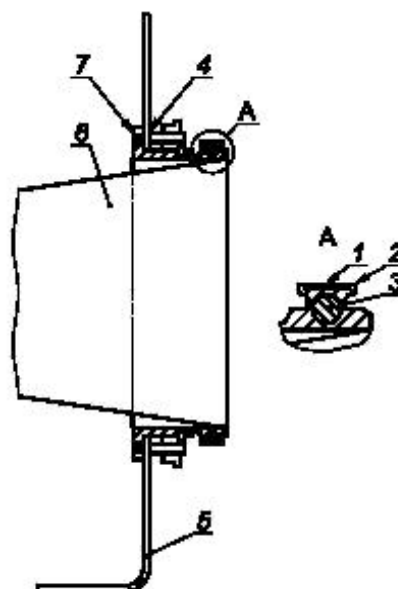
Рисунок С.1 — Перчаточный порт и перчаточный узел
