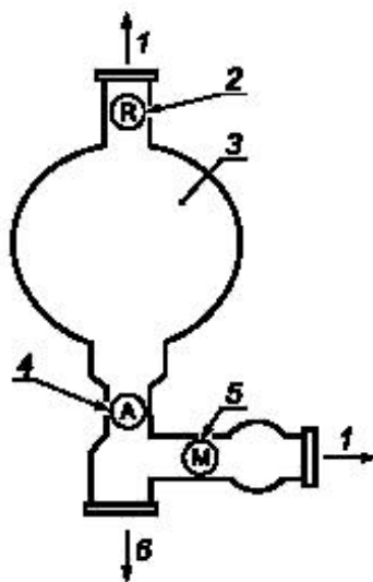
1 — направление в атмосферу, 2 — клапан В; 3 — резиновая груша; 4 — клапан А; 5 — клапан М; 6 — направление к трубке Парджо
